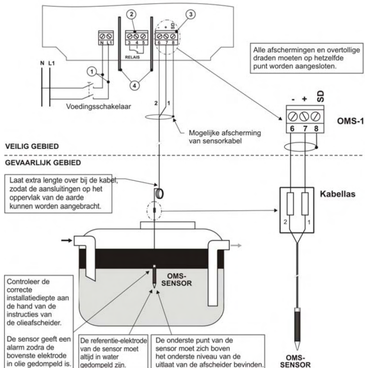
Afbeelding 3. Installatie van alarmtoestel OMS-1
