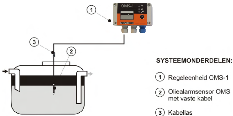
Afbeelding 1. Bewaking olieafscheider met alarmtoestel OMS-1
