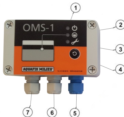
Afbeelding 2. Functies van regeleenheid OMS-1
